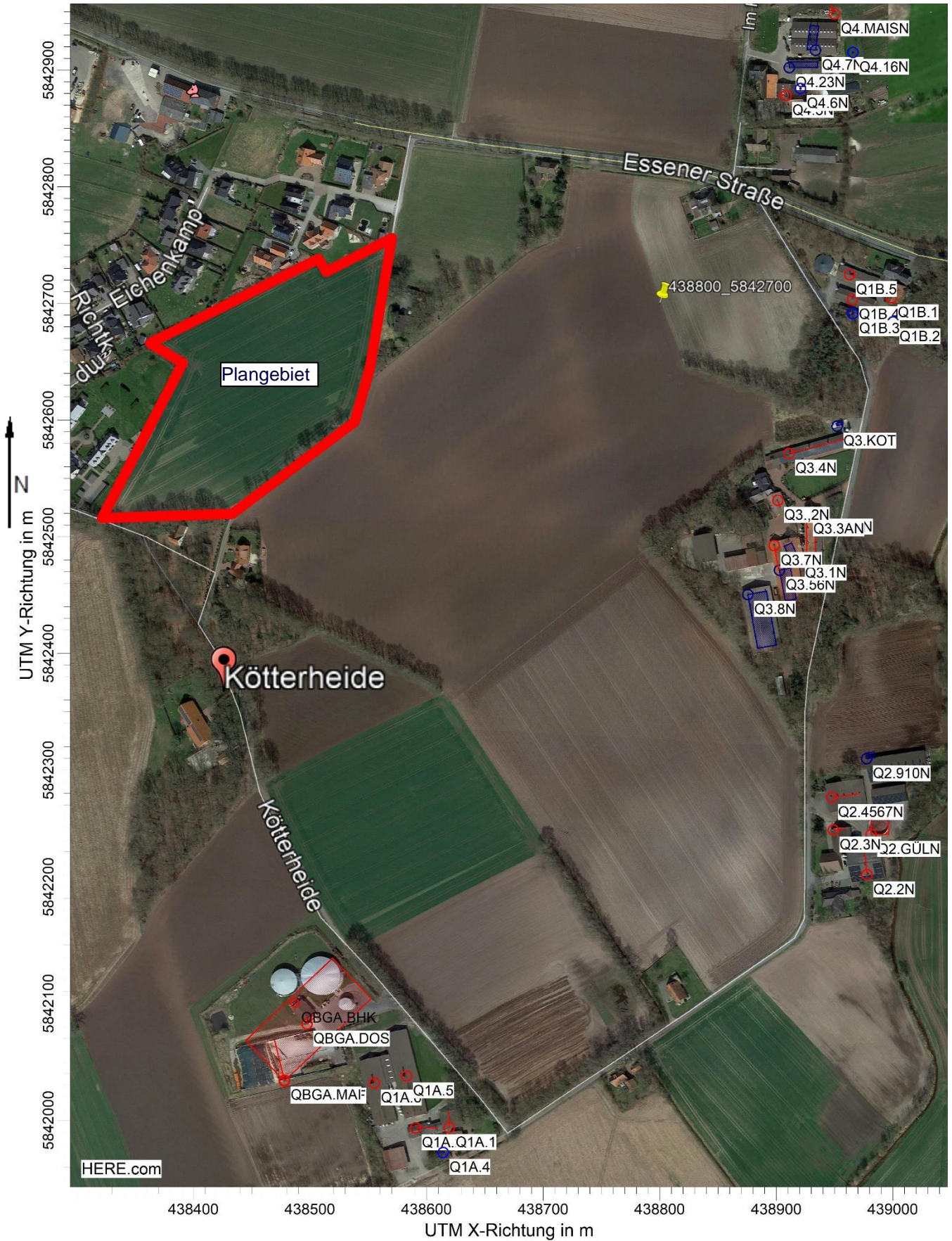
Abbildung 1: Lageplan Geruchsquellen; Zuordnung auf Seite 4 Plangebiet
